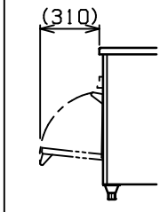
オ - プン扉開時寸法
