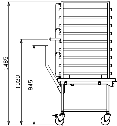
組図 RHM - C + RHM - R9
