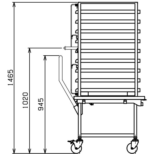
組図 RHM - C + RHM - R 9
